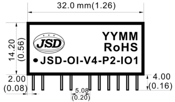
电压输入/电流输出 (V/I转换)
