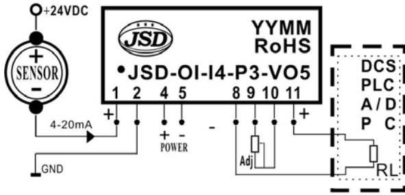
电流输入/电压输出 (I/V转换)
