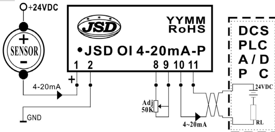
电流输入/电流输出 (无源隔离调理器)
