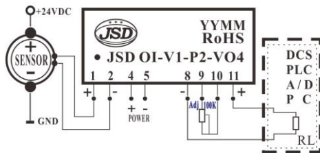
电压输入/电压输出 (V/V隔离)
