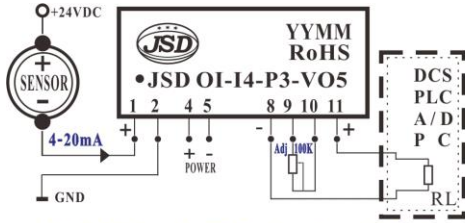
电流输入/电压输出 (I/V转换)
