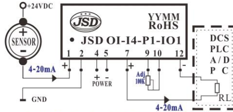
电流输入/电流输出 (I/I隔离)
